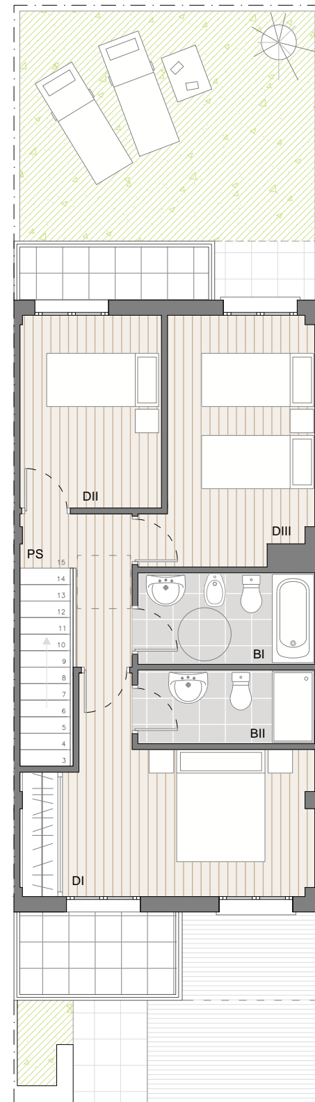
PLANTA PRIMERA
