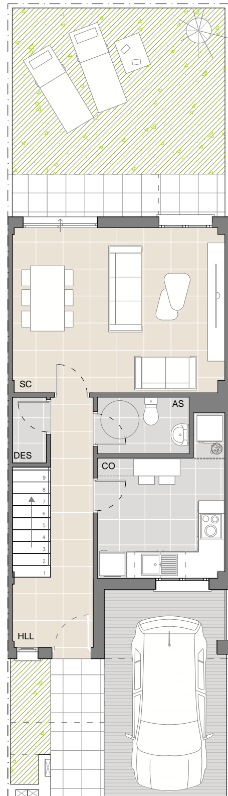
PLANTA BAJA
