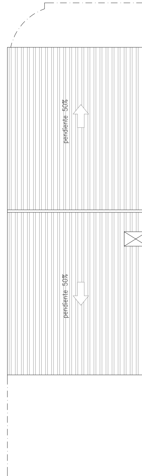
PLANTA DE CUBIERTAS
